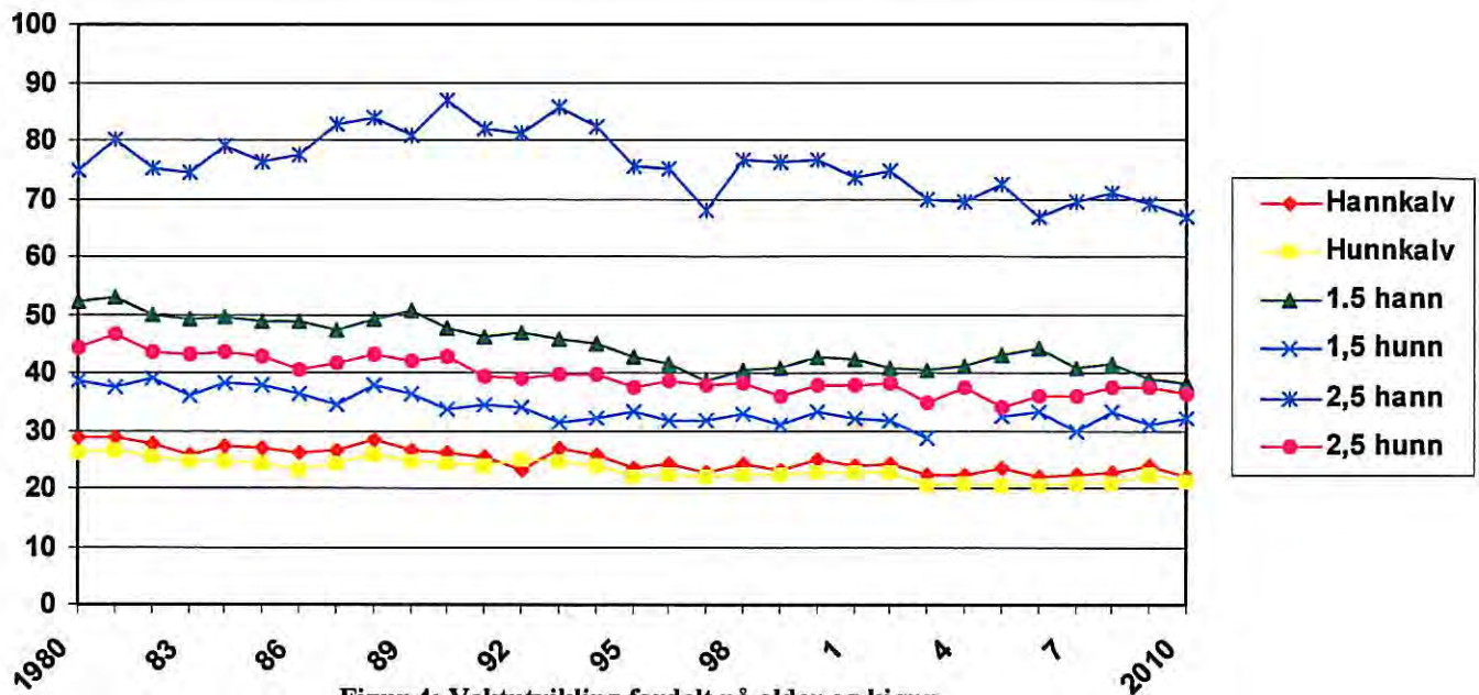
Figur 4: Vektutvikling fordelt på alder og kjønn
