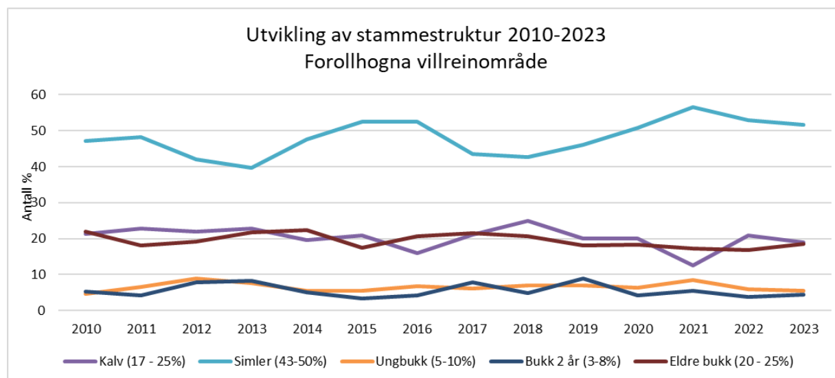
Figur 6 Utvikling av stammestruktur (strukturtellinger) 2010-2023
